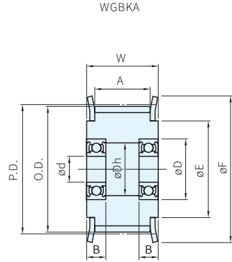
兩端軸承型
